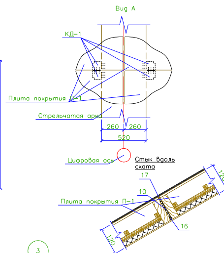
Поз. Обозначение Наименование Кол-во на 1 Кол-во на 1 объект Плита покрытия П-1 506 Сборочные единицы плиты П-1 Каркас ДК-1 1 506 1 ГОСТ 3916-69* Фанерный лист ФСФ -1500х3980 1 506 2 ГОСТ 3916-69* Фанерный лист ФСФ -1490х3980 10 506 3 ГОСТ 8486-86Е Прижимные бруски продольные 25х25х269 27 13662 4 ГОСТ 8486-86Е Прижимные бруски поперечные 25х25х139 18 9108 5 ГОСТ 15588-70* Утеплитель пенополистирол 439х269х5, q=150 кг/м² 9 4554 Каркас ДК-1 Сборочные единицы каркаса ДК-1 6 ГОСТ 8486-86Е Поперечное ребро ? 43х104х1490 2 1012 7 ГОСТ 8486-86Е Поперечное ребро ? 43х104х1490 2 1012 8 ГОСТ 8486-86Е Продольное ребро ? 43х104х3980 2 1012 9 ГОСТ 8486-86Е Продольное ребро ? 43х104х3980 2 1012 10 ГОСТ 16381-77* Минеральный войлок 11 ГОСТ 8486-86Е Разделительный брус поперечный 20х20, l=1500 460 12 Шуруп ?4, l=40 мм 24 12144 13 Шуруп ?6, l=60 мм 24 12144 Крепежная деталь КД-1 14 2 уголка стальные 75х75х5, l=100 мм между ? 75х75х5, l=100 мм 4 2024 15 Слой пергамина на мастике или полиэтиленовая пленка 16 Пароизол 17 ГОСТ 8486-86Е Разделительный брус продольный 20х20, l=3980 506 18 ГОСТ 8486-86Е Разделительный брус поперечный 20х20, l=1250 400
