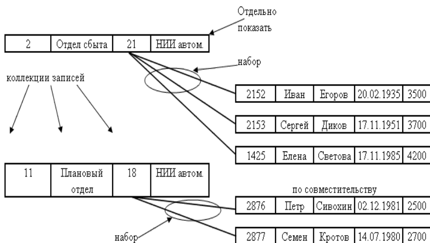
Рис.8. Сетевая модель данных
