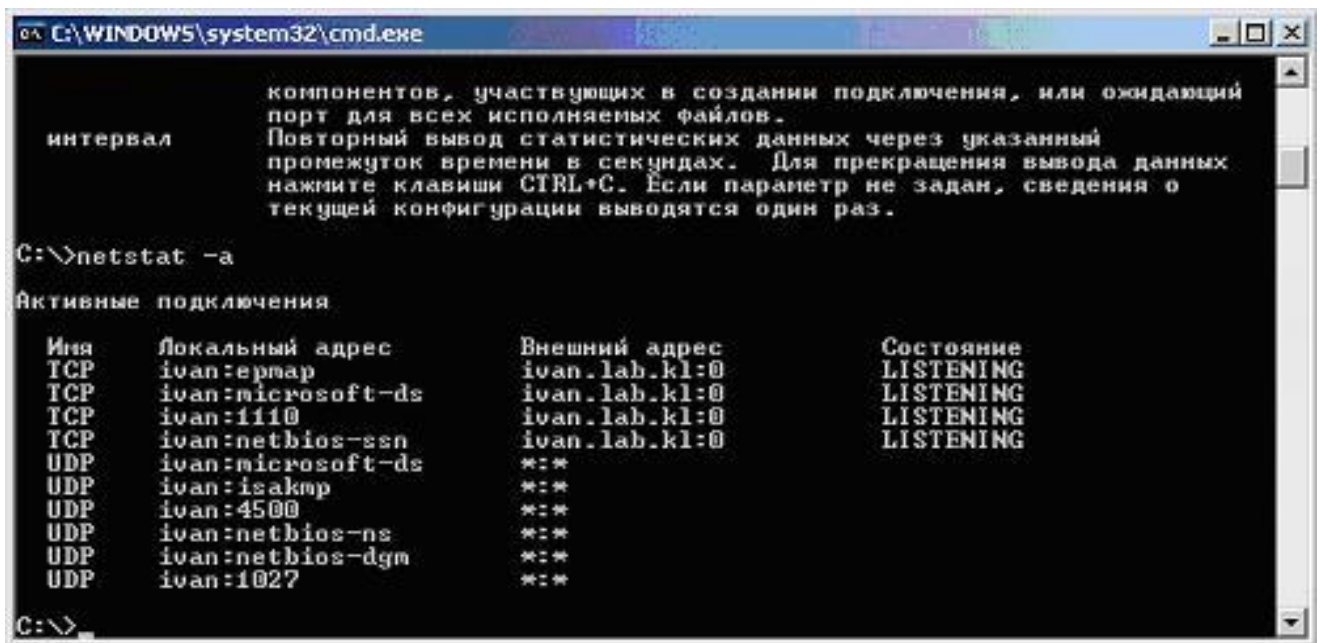
Рис. 11. Окно утилиты Командная строка.
