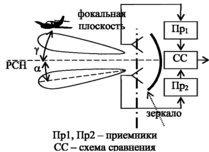
Рис. 35. Структурная схема многоканального (моноимпульсного) измерителя угловых координат
