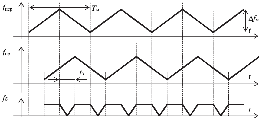
Рис. 32. Частотный метод измерения дальности неподвижной цели: \Delta f_M – девиация частоты; T_M = 1/F_M – период модуляции излучаемого колебания
