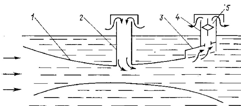
Рис.46. Схема объемного насоса: 1 – профилированный корпус; 2 – шахта воздухозаборника; 3 – воздухосборник; 4 – выхлопная шахта; 5 – воздушная турбина с электрогенератором.
