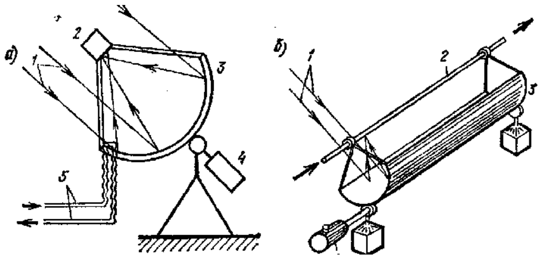
Рис.7. Концентрирующие гелиоприемники: а – параболический концентратор; б – параболоцилиндрический концентратор; 1 – солнечные лучи; 2 – тепловоспринимающий элемент (солнечный коллектор); 3 – зеркало; 4 – механизм привода системы слежения; 5 – трубопроводы, подводящие и отводящие теплоноситель.
