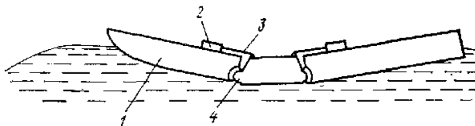
Рис.40. Вариант выполнения контурного плота Коккерелла: 1 – колеблющаяся секция; 2 – преобразователь; 3 – тяга; 4 – шарнир.
