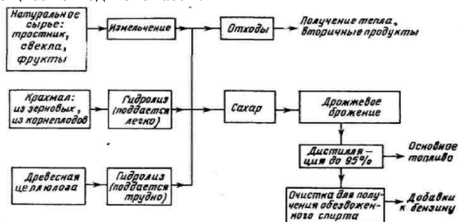
Рис.55. Производство этанола
