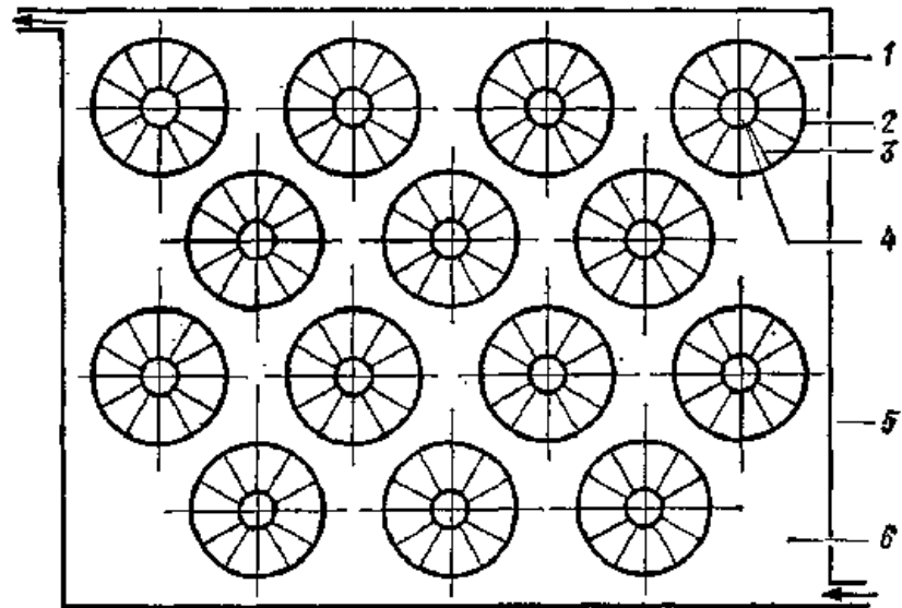
Рис.18. Теплообменник с оребренными кольцевыми каналами для аккумуляции энергии с использованием теплоты фазового перехода: 1 – элемент теплообменного блока; 2 – термоаккумулирующее вещество; 3 – продольное ребро; 4 – горячий теплоноситель; 5 – резервуар (кожух); 6 – холодный теплоноситель для разрядки.
