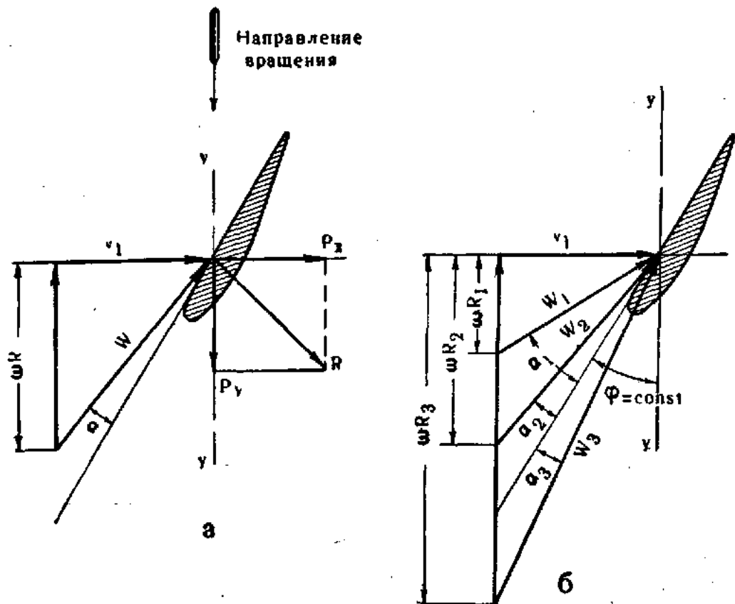
Рис.26. а – схема действия сил воздушного потока на элемент лопасти; б – графическое изображение относительного потока, набегающего на элементы лопасти, расположенные на разных радиусах ветроколеса.
