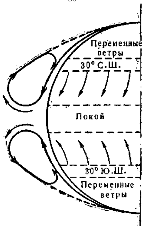
Рис.19. Схема общей циркуляции земной атмосферы
