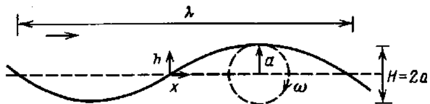
Рис.37. Характеристики волны.
