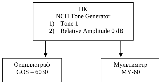
Рис. 21. Структура лабораторной установки
