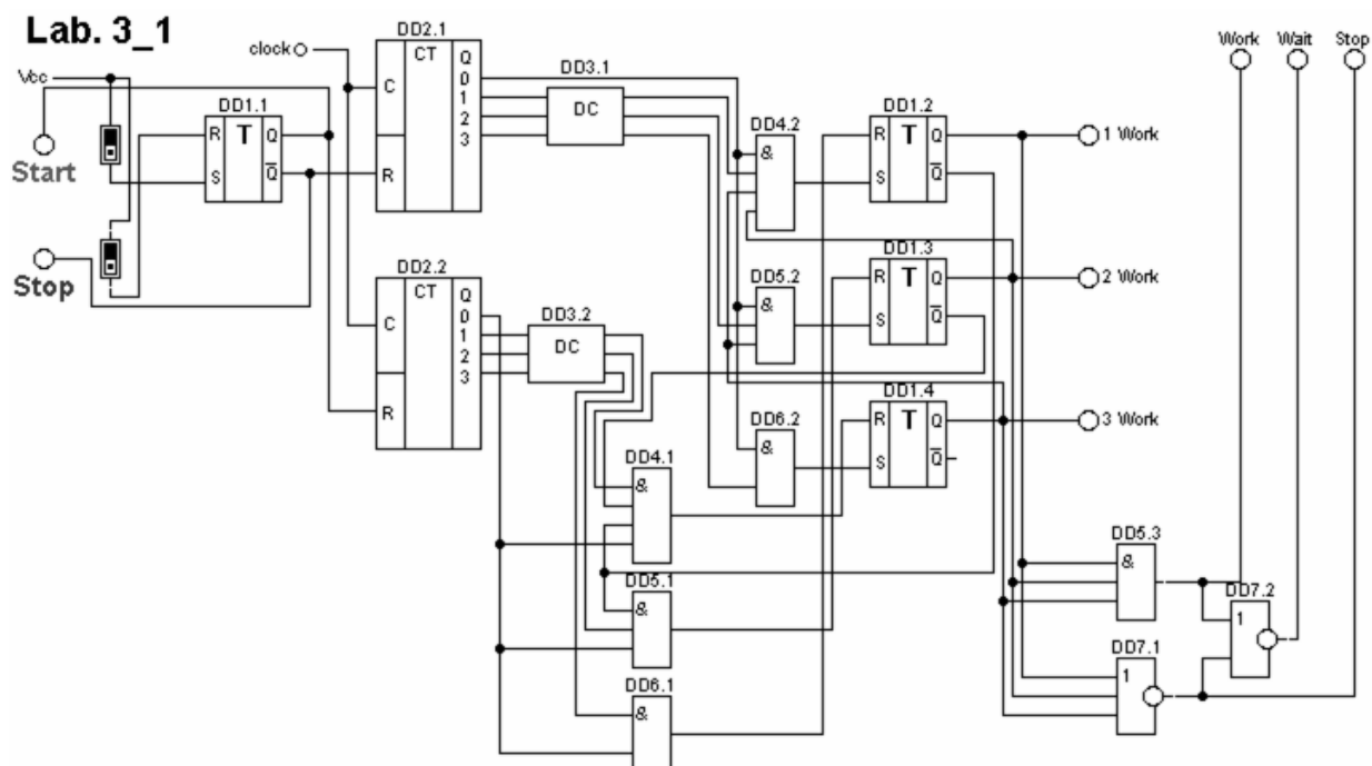
Рис. 20. Принципиальная схема управления транспортёром
