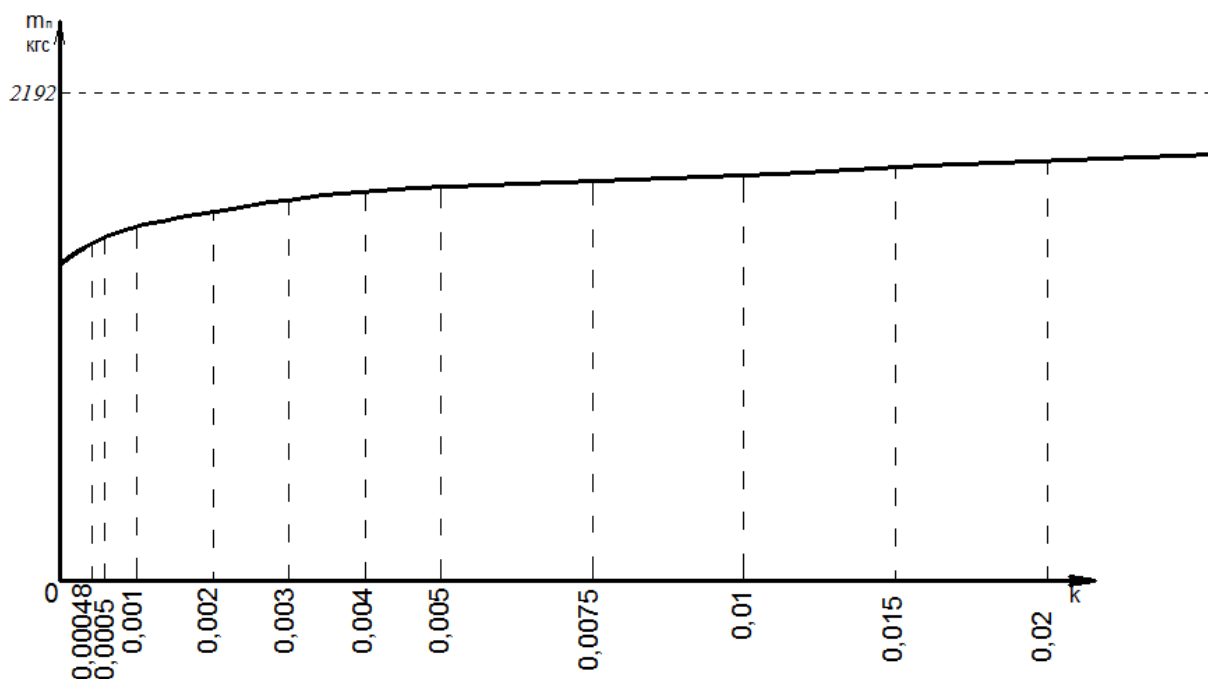
Рис. 18. График зависимости массы m_{\pi} \left( \frac{l}{6} \right) = f(k) .
