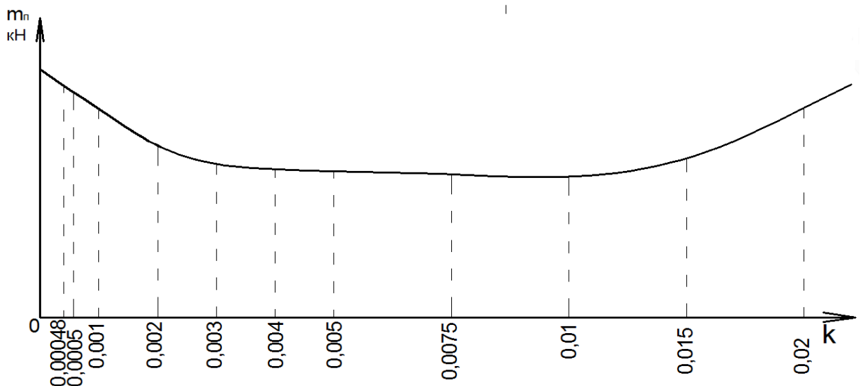
Рис. 17. График зависимости массы m_n \left( \frac{l}{3} \right) = f(k) .
