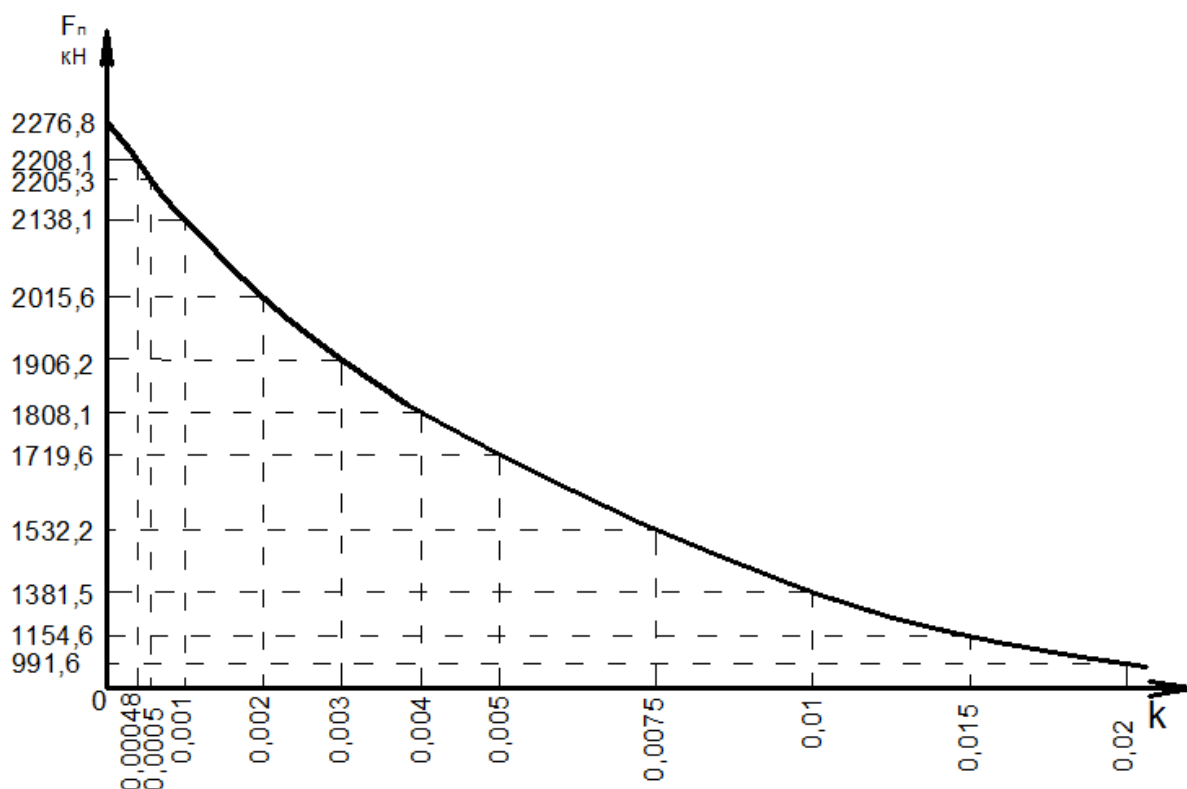
Рис. 16. График зависимости усилий F_n = f(k) .
