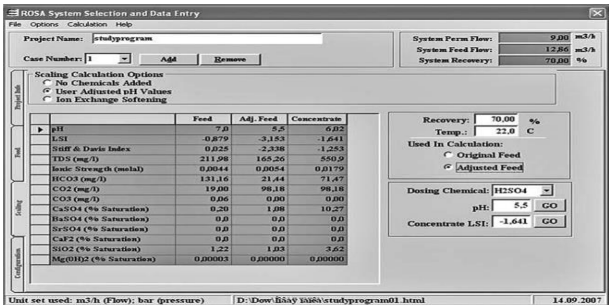
Рисунок 2. Вкладка Scaling .
