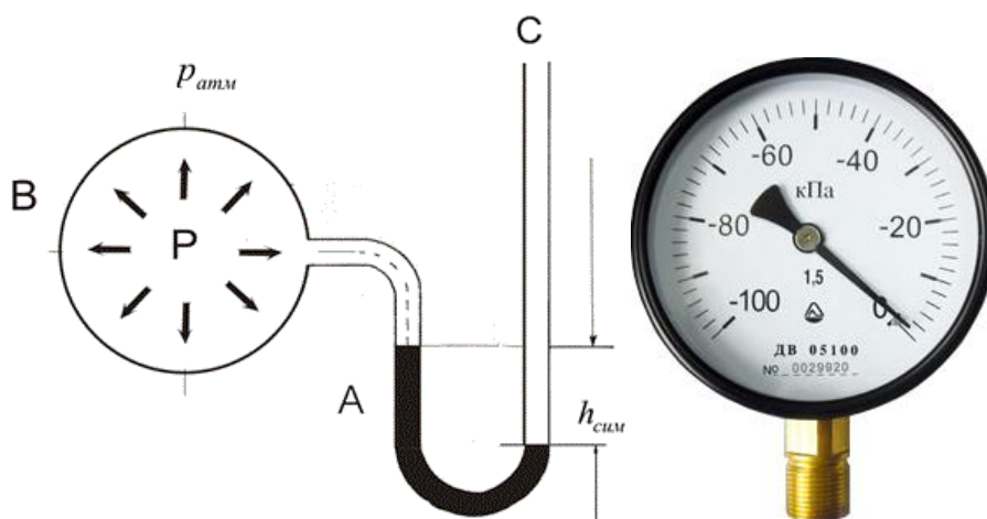
Рис. 3. Вакуумметр
