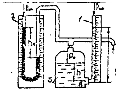
Рис. 7. Схема экспериментальной установки.
