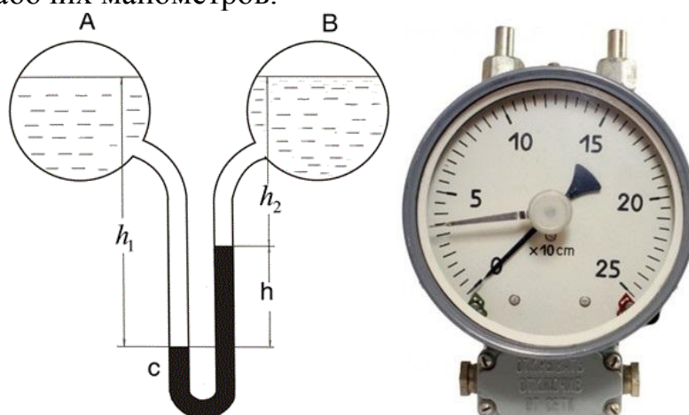
Рис. 6. Дифференциальный манометр.
