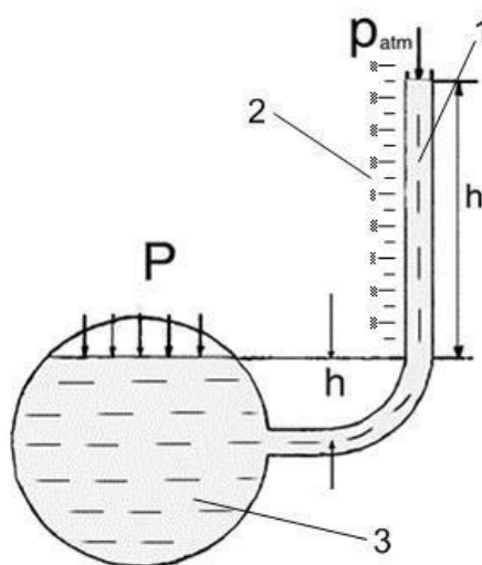
Рис. 1. Пьезометр
