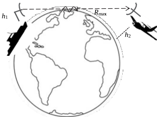
Рис. 6. Влияние сферичности Земли на дальность действия РТС
