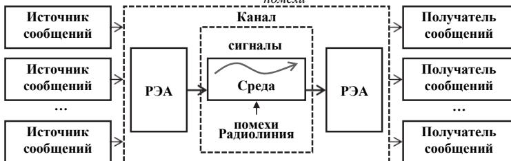
Рис. 10. Структура РТС ПИ
