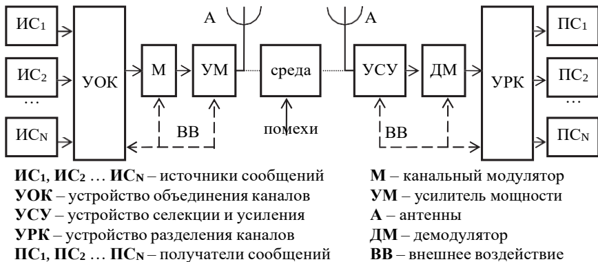
Рис. 1. Обобщенная структурная схема многоканальной системы передачи информации
