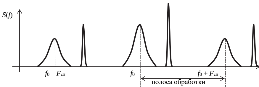
Рис. 42. Спектр отраженного сигнала
