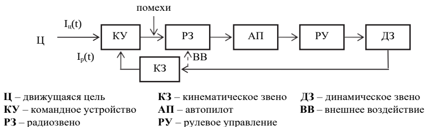
Рис. 2. Структурная схема системы радиопередачи зенитной ракетой
