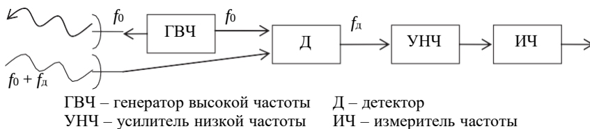
Рис. 38. Структурная схема измерителя радиальной скорости
