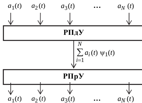
Рис. 11. Обобщенная структурная схема многоканальной системы
