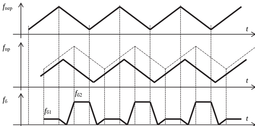
Рис. 33. Частотный метод измерения дальности подвижной цели
