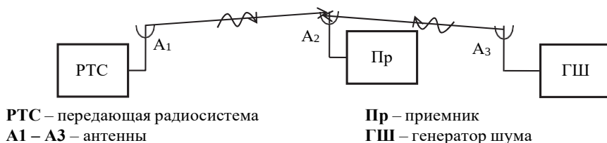
Рис. 4. Структурная схема системы радиопротиводействия
