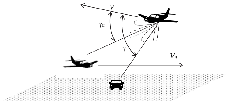
Рис. 39. К принципу работы импульсно-доплеровских РЛС
