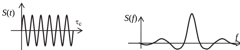
Рис. 21. Простой радиосигнал: временное и частотное представление
