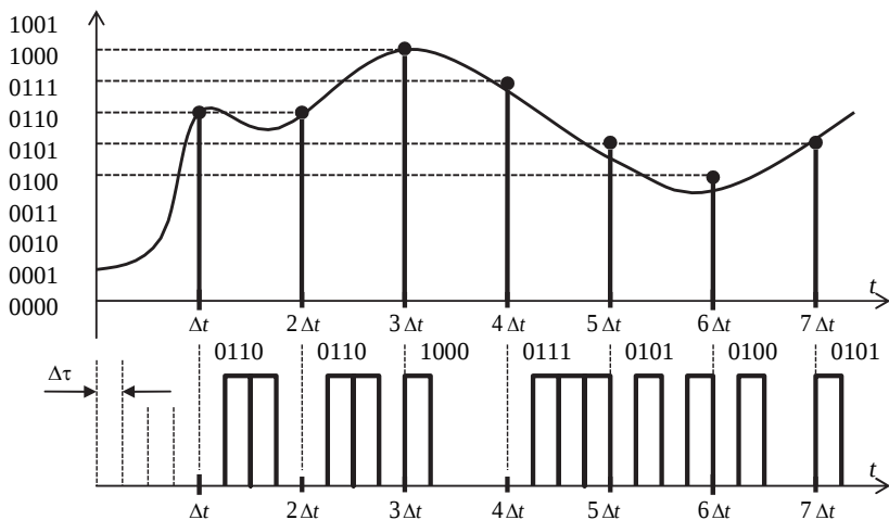
Рис. 18. Принцип формирования сигнала в системе с ИКМ
