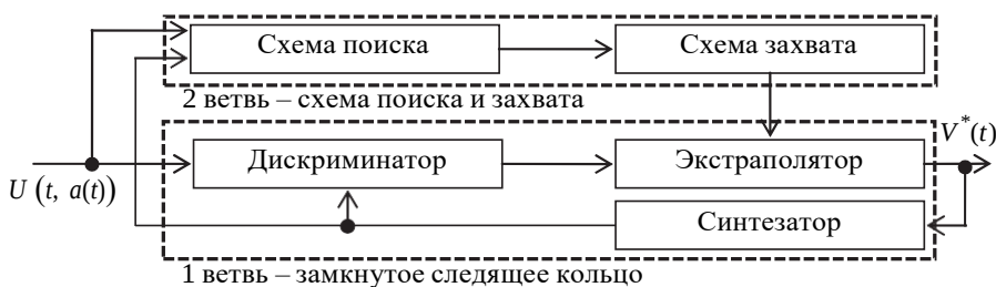
Рис. 45. Структурная схема слеящего измерителя
