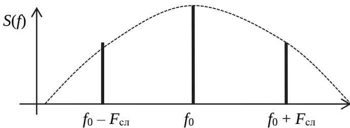
Рис. 41. Спектр последовательности зондирующих импульсов
