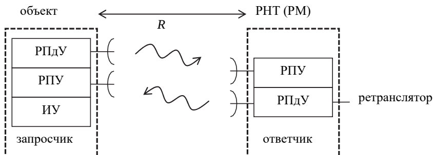
Рис. 57. Структурная схема круговой РНС
