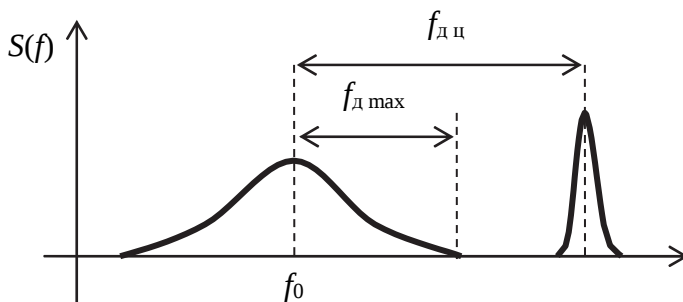
Рис. 40. Спектр наблюдаемого сигнала
