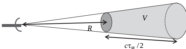
Рис. 8. ЭПР объемно-распределенной цели
