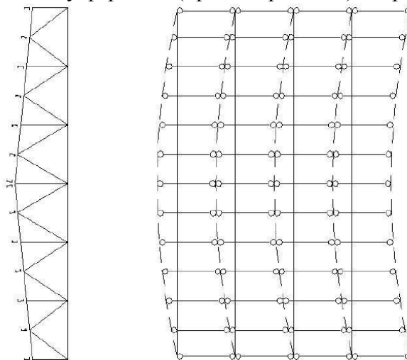
Рис. 17.3. Потеря устойчивости верхних поясов ферм в покрытии без связей.
