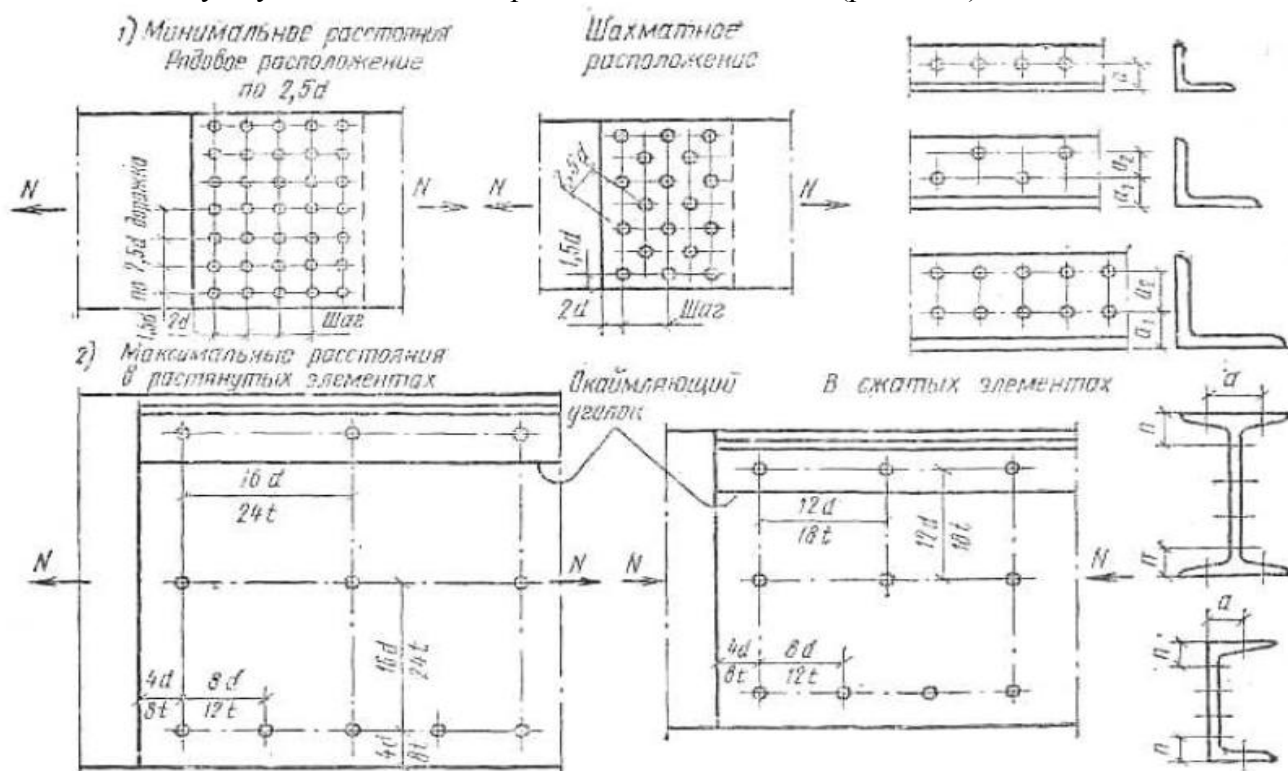
Рис. 10.4. Размещение отверстий.
