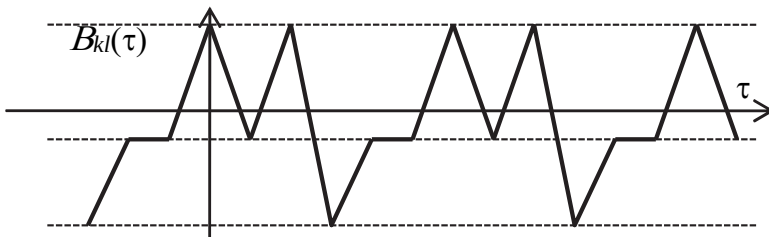
Рис. 27. Пример трехуровневой ВКФ двух M -последовательностей, образующих код Голда
