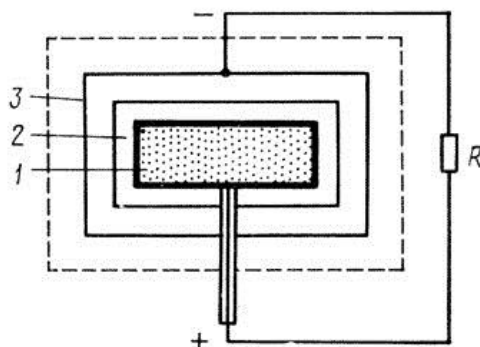
Рис. 5.8. Установка прямого преобразования ядерной энергии в электрическую: 1 – \beta -радиоактивный излучатель; 2 – металлическая; ампула; 3 – металлический сосуд
