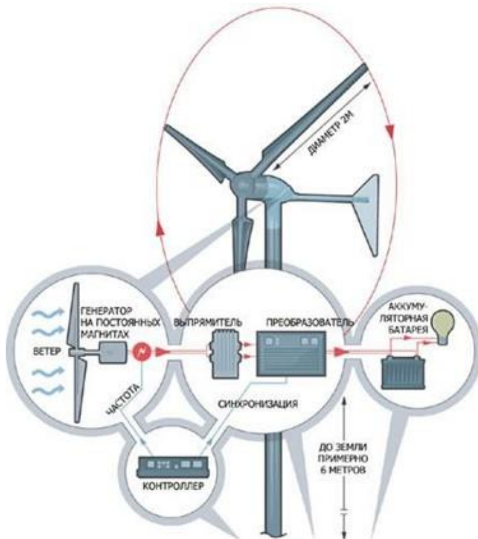
Рис. 4.7. Ветровая турбина
