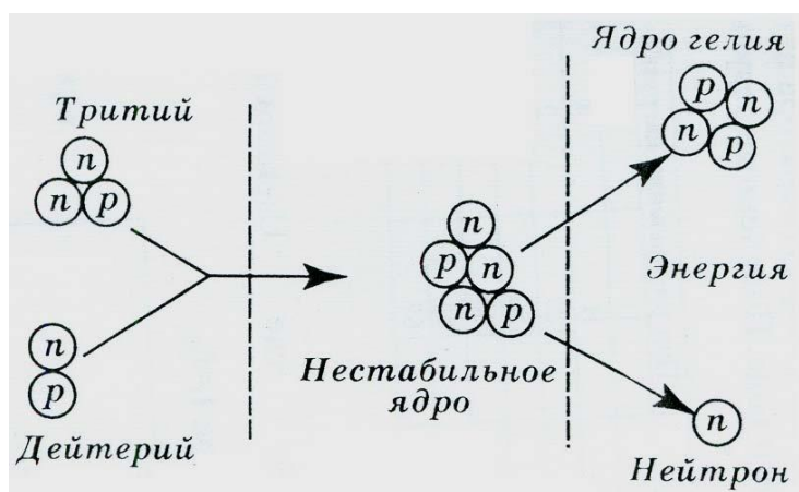
Рис. 5.1. Реакция синтеза изотопов водорода – дейтерия и трития
