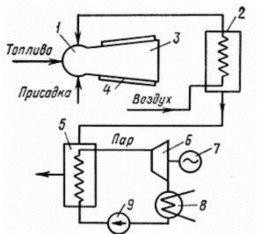
Рис. 5.6. Принципиальная схема МГД-генератора с паросиловой установкой:
