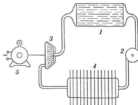
Рис. 5.9. Принципиальная схема радиоизотопного турбогенератора
