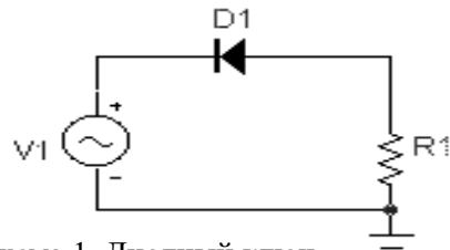
Схема 1. Диодный ключ. V1 – 80 Гц, 6В D1 – 1N3017A; R1 – 1k
