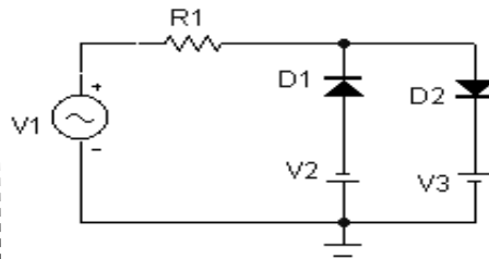
Схема 2. Двухсторонний ограничитель. V1 – 30 Гц, 6В D1, D2 – 1N3017A; V1, V2 – 4В; R1 – 1k
