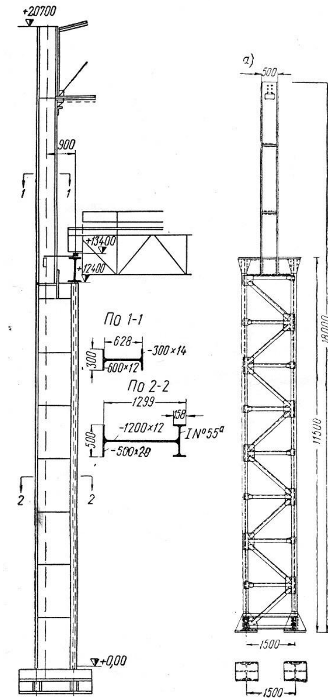
Пример наружной сплошной ступенчатой колонны
