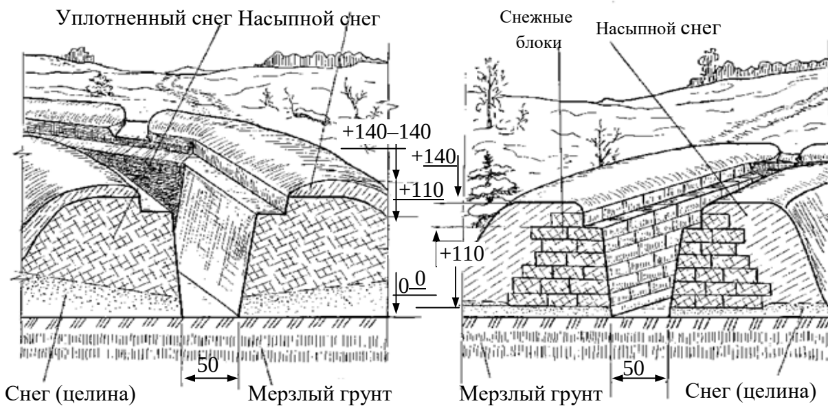
Рис. 6.20. Профили траншей, устраиваемых зимой: а – при глубине промерзания 10–15 см или небольшом снежном покрове; б – при большой глубине промерзания и снежном покрове до 1 м; в, г – при глубине снежного покрова более 1 м
