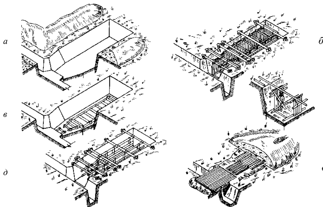
Рис. 6.21. Порядок сборки убежища безврубочной конструкции: а - подготовка котлована; б - монтаж нижней опорной рамы; в - монтаж верхней опорной рамы; г, д - монтаж заборки стен; е - укладка покрытия и обсыпка
