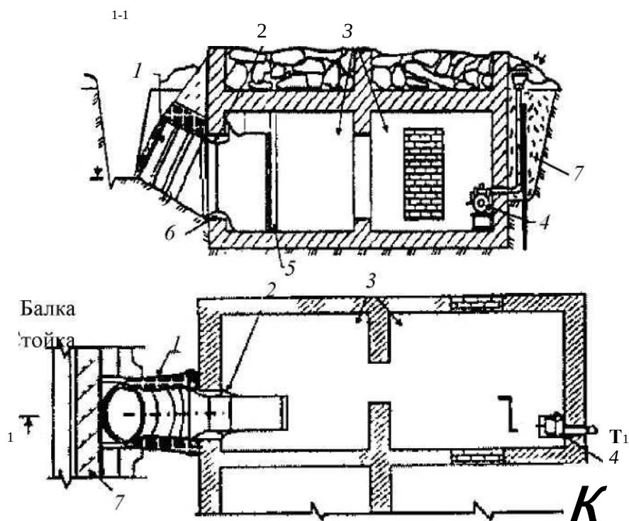
Рис. 6.31. Убежище в подвальном помещении, оборудованное входом ЛАЗ-2:
