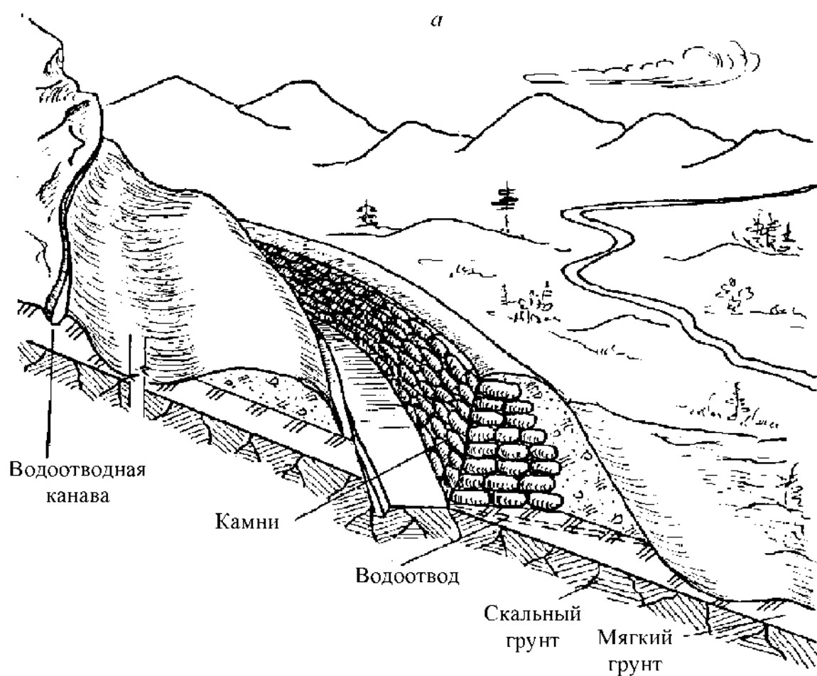
Рис. 6.19. Сооружения открытого типа в горной местности: а - окоп для танка в горной местности; б - профиль стрелковых окопов и траншей
