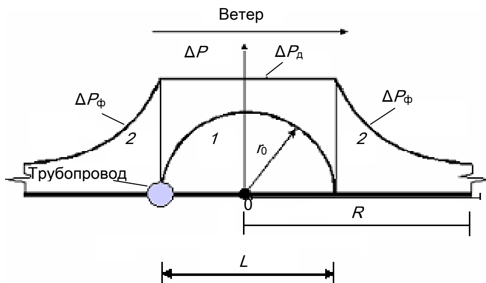
Рис. 3.15. Расчетная схема к определению давлений при аварии на газопроводе: \Delta P_d – давление в зоне детонации; \Delta P_\phi – давление во фронте воздушной ударной волны; r_0 – радиус зоны детонации; R – расстояние от расчетного центра взрыва; 0 – центр взрыва; 1 – зона детонации; 2 – зона воздушной ударной волны ( R > r_0 )
