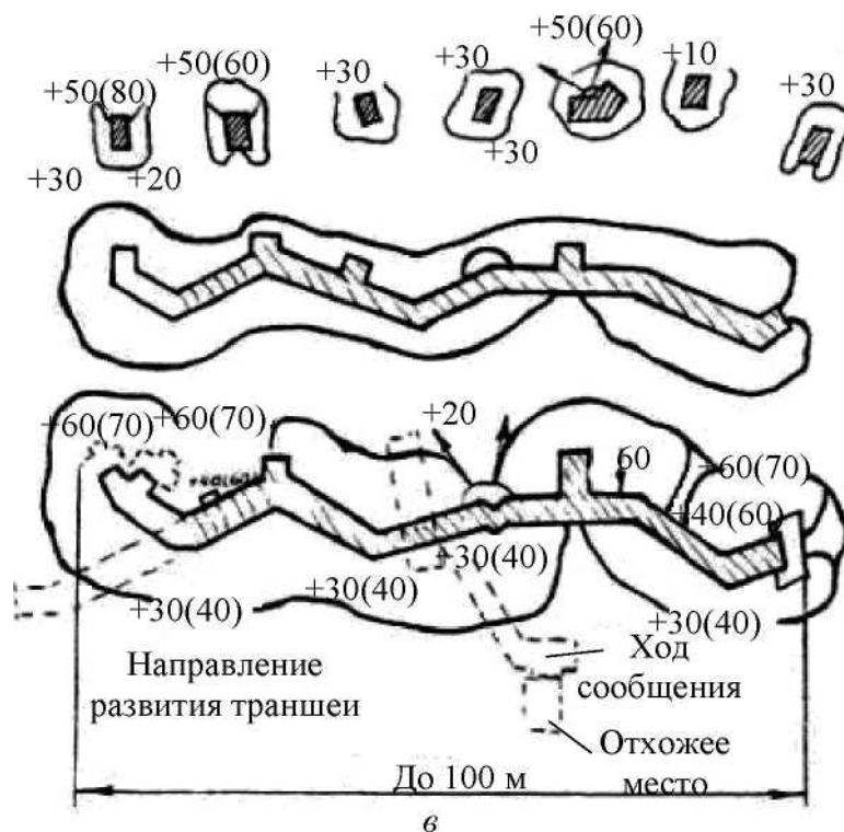
Рис. 6.6. Стрелковые окопы: а - для стрельбы из автомата стоя; б - для стрельбы из пулемета стоя; в - последовательность развития окопа на отделение
