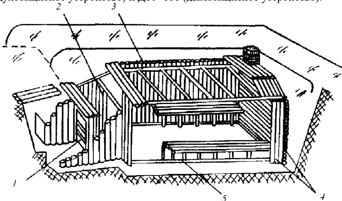
Рис. 6.11. Убежище безврубочной конструкции: 1 - дверной блок БД-60; 2 - герметическая дверь; 3 - верхняя опорная рама; 4 - забирка стен; 5 - нижняя опорная рама
