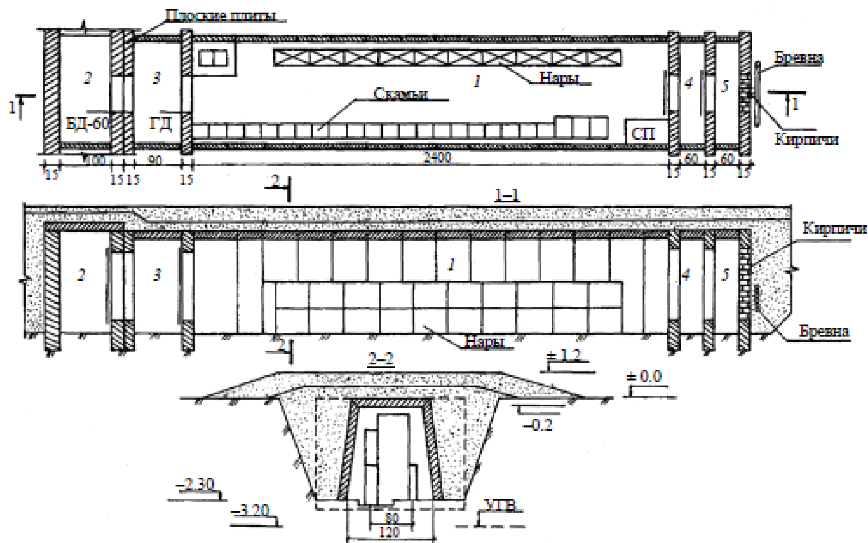
Рис. 5.5. Схема быстровозводимого убежища из трехпанельных плит типа «Фара»: 1 – помещение для укрываемых; 2 – вход; 3 – тамбур; 4 – фильтровая; 5 – расширительная камера
