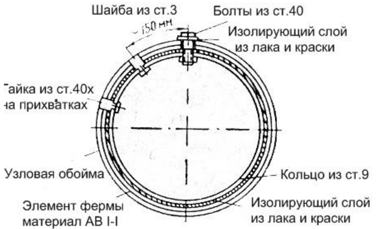
Разрез 1-1
