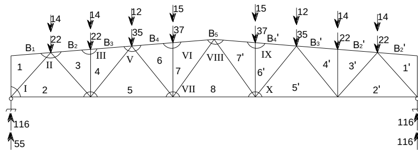
рис 6.4. Расчетная схема при постоянной и снеговой нагрузках
