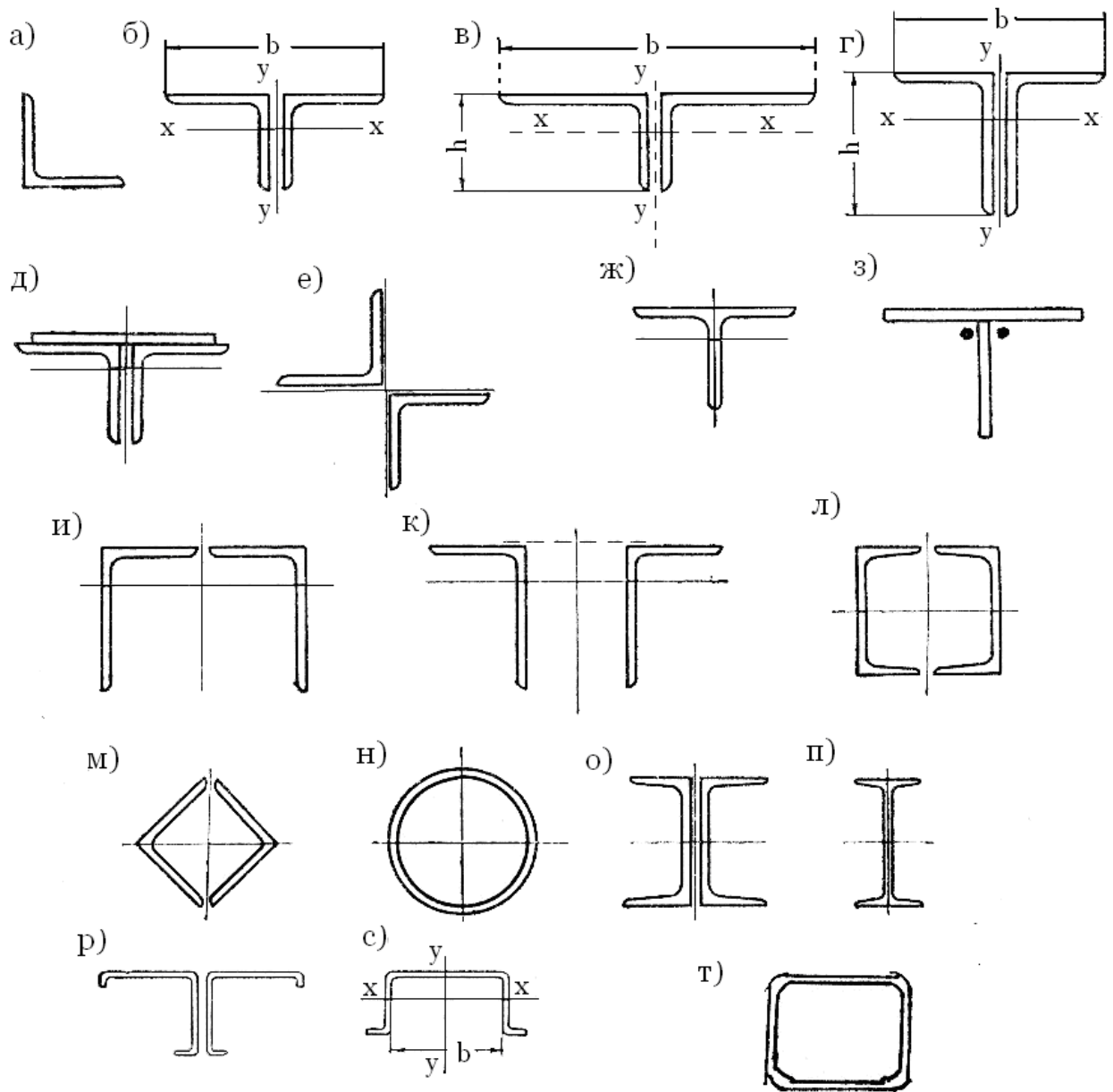
Типы сечений стержней легких ферм
