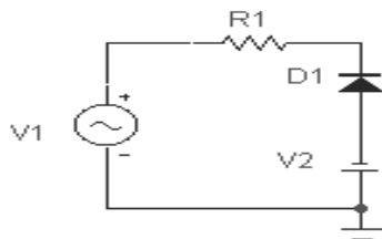
Схема 2. Односторонний ограничитель.
