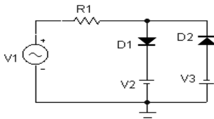
Схема 2. Двухсторонний ограничитель.
