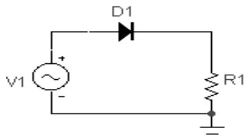
Схема 1. Диодный ключ.
