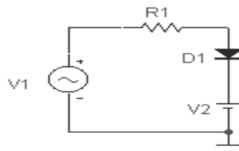
Схема 2. Односторонний ограничитель.
