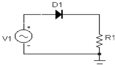
Схема 1. Диодный ключ.
