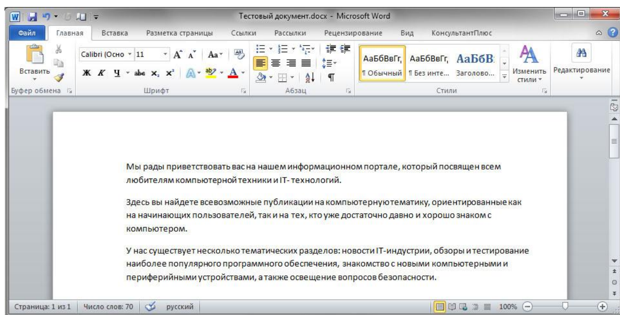
Рисунок 13. Вариант текста
