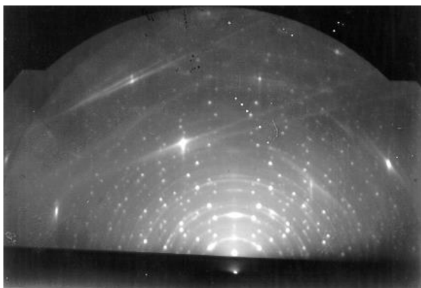
Рис. 3.16. Электронограмма на отражение от пленки оксида вольфрама на 50 мин. отжига в кислороде ( T=650^\circ\text{C} , p=1,33 Па) исходной эпитаксиальной пленки \text{WO}_2 (см. рис. 3.12).
