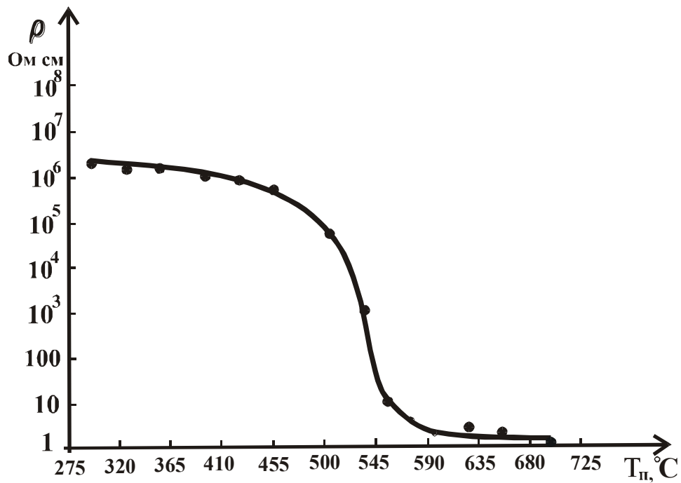
Рис.4.1. Зависимость удельного сопротивления пленок от температуры подложки.
