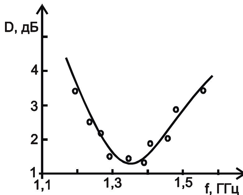
Рис. 4.9. Частотная зависимость потерь на двойное преобразование пленочного ZnO-преобразователя продольных волн.
