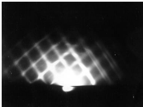
Рис. 3.15. Электронограмма на отражение от пленки оксида вольфрама после отжига в кислороде ( T=650^\circ\text{C} , p=1,33 Па) исходной эпитаксиальной пленки \text{WO}_2 (см. рис. 3.12) в течение 20 мин.
