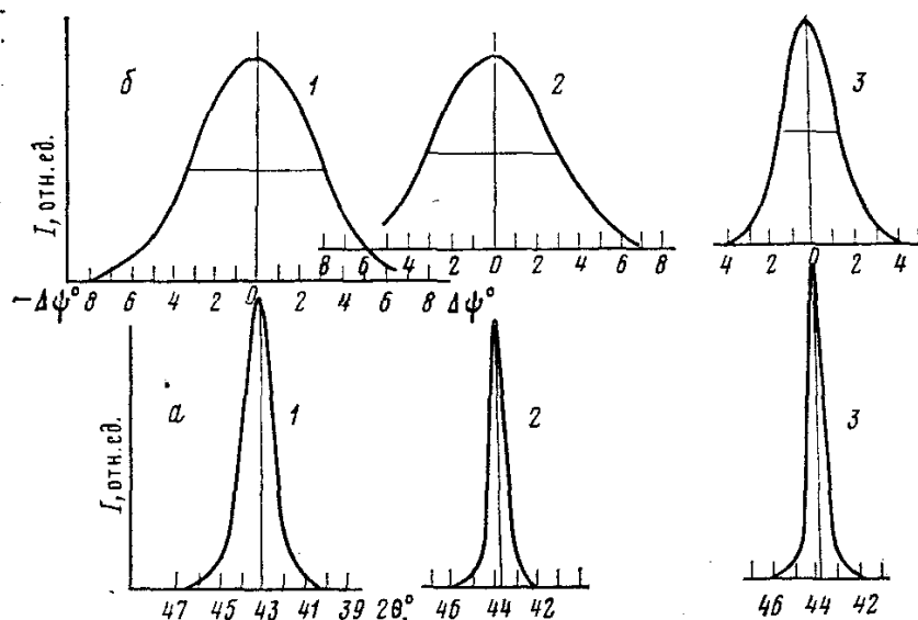
Рис. 1.9. Фрагменты дифрактограмм (а) и кривые качения (б) свеженапыленной (1) и отожженных (2,3) пленок оксида цинка толщиной 2 мкм, полученных при T_n=473 К, v_n \leq v_{гр} и расстоянии мишень-подложка 0,10 (1,2) и 0,08 м (3): а) кривая 1: L=26 нм, (\Delta d/d)_2=0,86\% , (\Delta d/d)_1=1,2\% ; кривая 2: L=26 нм, (\Delta d/d)_2=0\% , (\Delta d/d)_1=0\% ; кривая 3: L=27 нм, (\Delta d/d)_2=0\% , (\Delta d/d)_1=0\% ; б) кривая 1: \theta=21^{\circ}35' , кривые 2,3: \theta=21^{\circ}35' .
