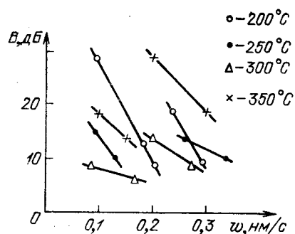
Рис. 1.12. Зависимость потерь на преобразование В в пленках ZnO от скорости их роста w и температуры подложки T_{\text{п}} .
