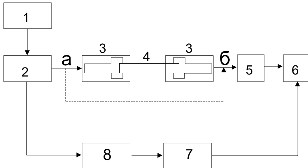
Рис.4.4. Блок схема изучения эффективности возбуждения гиперзвука в пленках ZnO. 1-источник питания; 2-генератор УВЧ; 3-объемные резонаторы; 4-звукопровод из Al_2O_3 с пленками ZnO на торцах; 5-супергетеродинный приемник; 6-осциллограф; 7-генератор импульсов; 8-модулятор.
