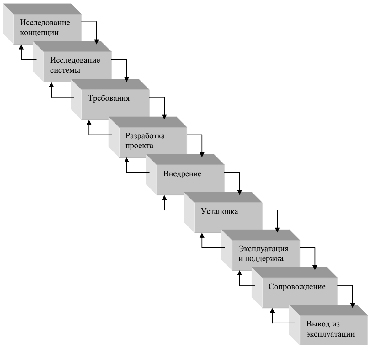
Рис. 4.4. Классическая каскадная модель с обратной связью.
