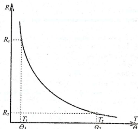
Рисунок 2.1 – График зависимости сопротивления полупроводникового резистора от температуры
