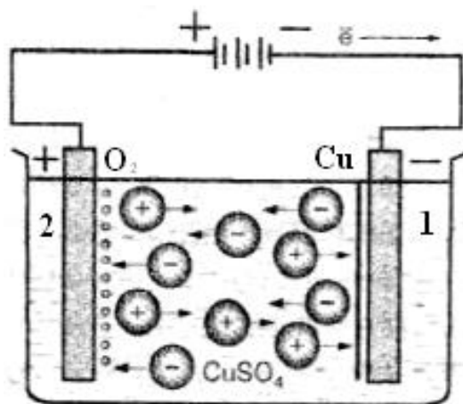
1 – катод, 2 – анод
