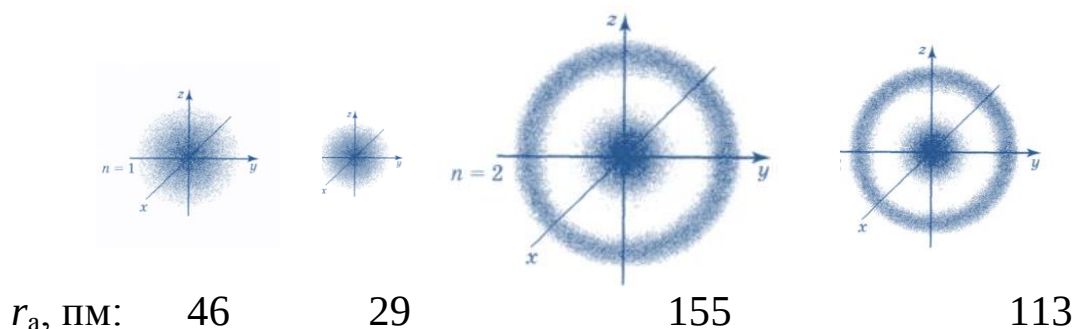
Рис. 25. Сечения 1s - и 2s -электронных облаков атомов водорода, гелия, лития и бериллия плоскостями, проходящими через их ядра
