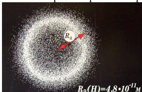
Радиус атома водорода
