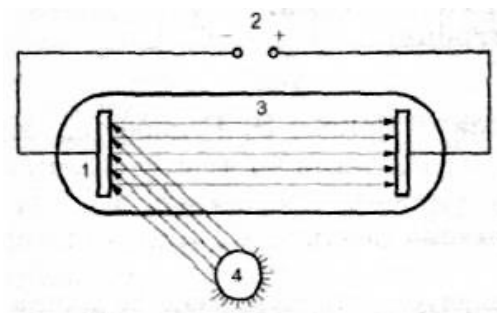
Рис. 3. Фотоэлектрический эффект
