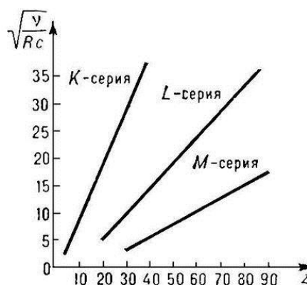
График закона Мозли
