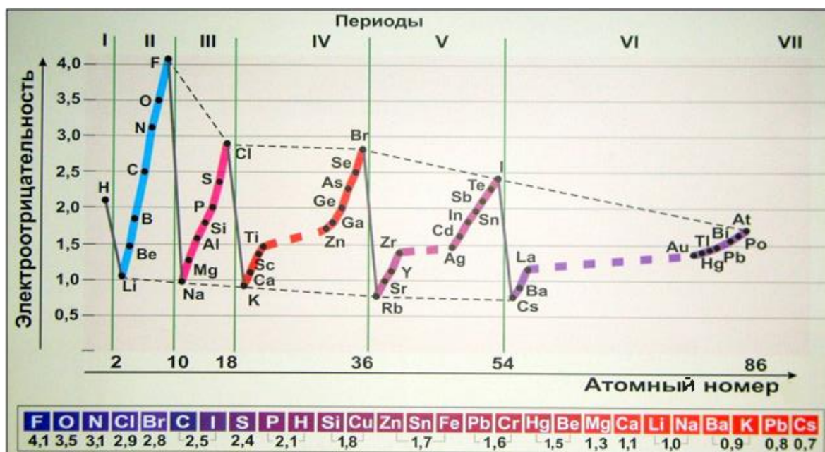
Рис. 40. Относительные электроотрицательности атомов химических элементов
