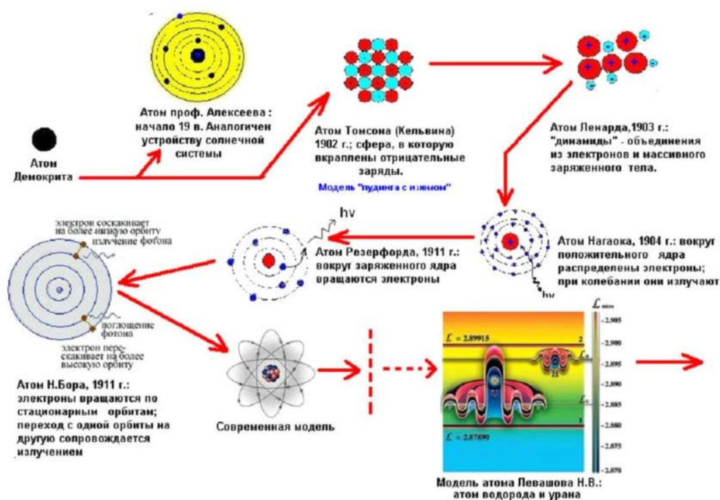
Рис. 7. Развитие представлений об атоме
