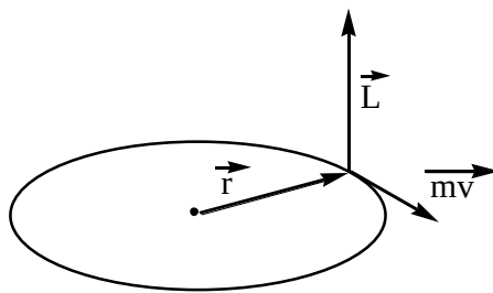
Рис. 18. Орбитальный момент количества движения
