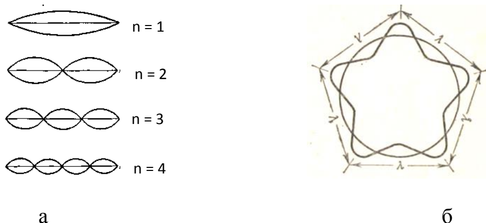
Рис. 16. Стоячие волны (а) в колеблющейся струне и (б) электронная волна в пределах атома ( n = 5 )
