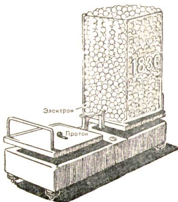
Рис. 12. Соотношение масс протона и электрона
