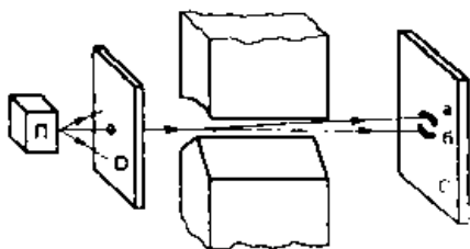
Схема опыта Штерна-Герлаха (1922) (доказательство наличия спина)
