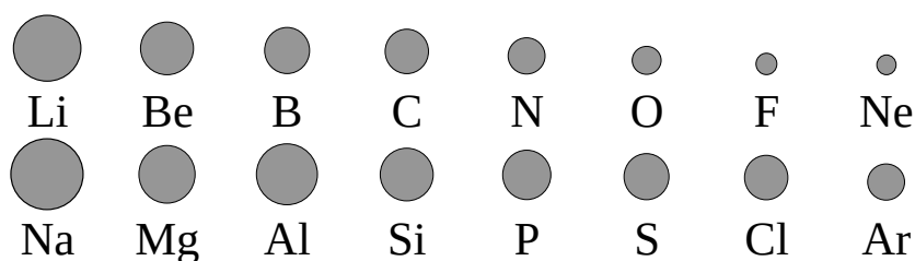
Рис. 35. Изменение радиусов атомов элементов второго и третьего периодов
