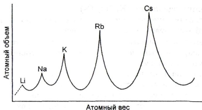
Рис. 28. Кривая атомных объёмов Мейера
