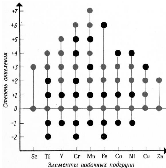
Рис. 42. Степени окисления, характерные для атомов 3d-элементов. (Наиболее часто встречающиеся степени окисления обозначены светлее)
