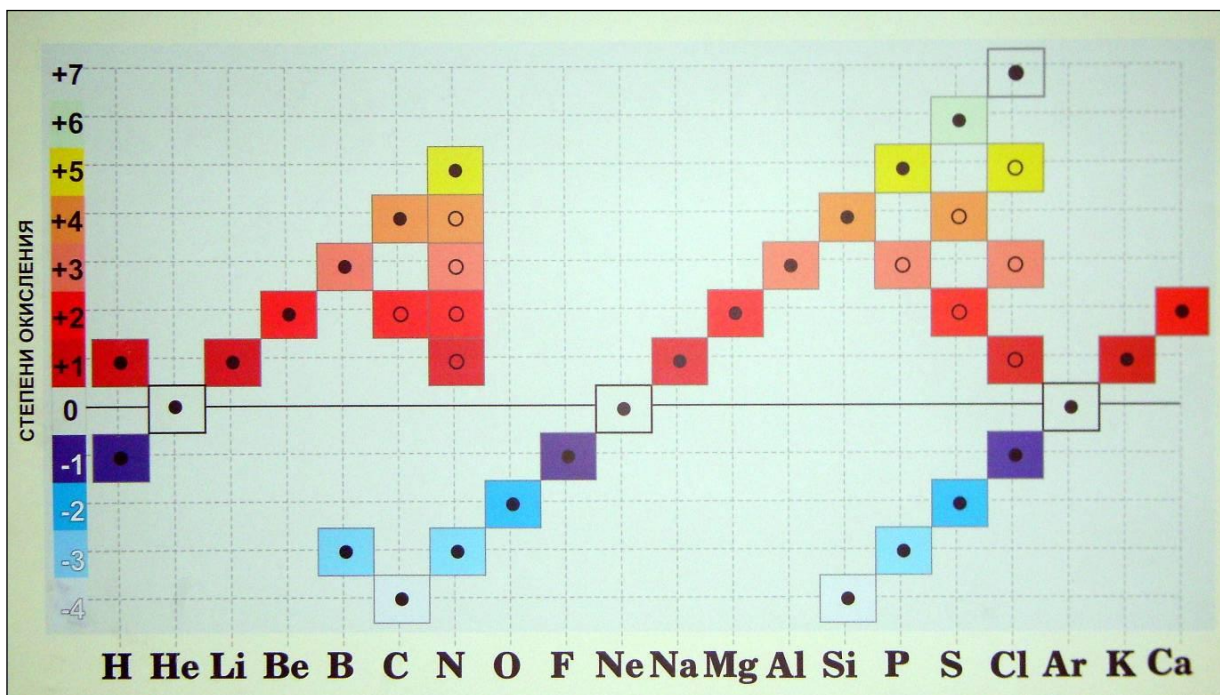
Рис. 43. Степени окисления атомов благородных газов и атомов химических элементов в сложных веществах
