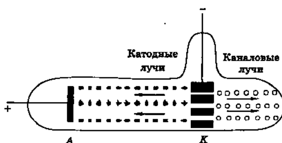
Рис. 2. Обнаружение каналových лучей
