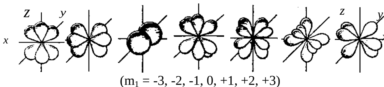
Рис. 20. Формы атомных орбиталей
