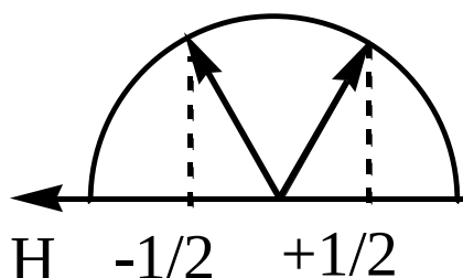
Рис. 22. Ориентации спинового момента электрона относительно внешнего магнитного поля
