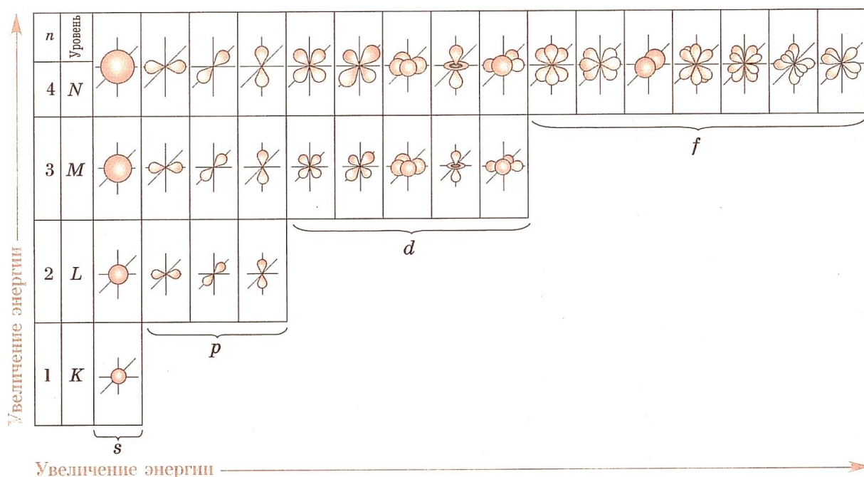
Форма и размер электронных орбиталей атомов элементов
