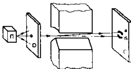
Рис. 21. Схема опыта Штерна-Герлаха
