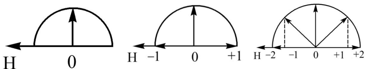
Расщепление энергетических уровней на подуровни
