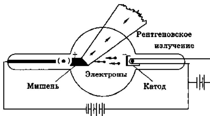
Рис. 4. Рентгеновская трубка
