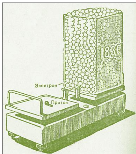
Соотношение масс протона и электрона
