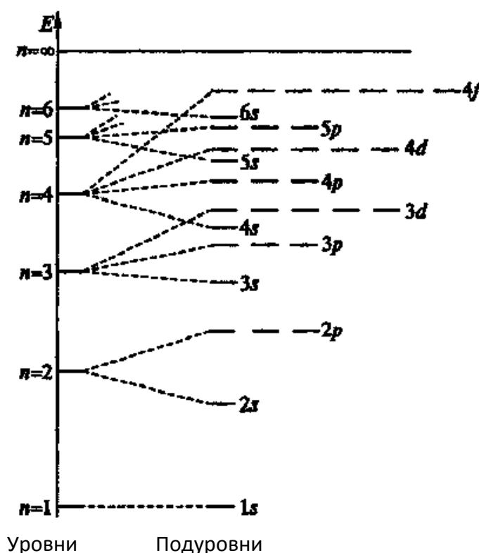
Рис. 24. Схема подразделения энергетических уровней атомов на подуровни
