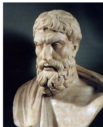
Эпикур 342-270 г. до н. э.
