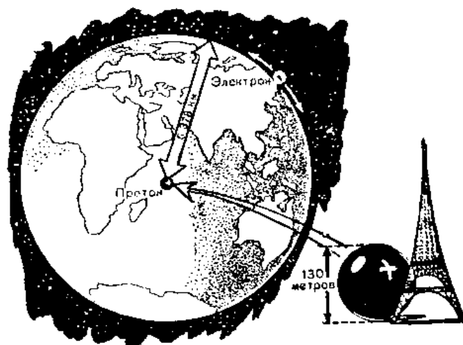
Рис. 13. Соотношение размеров ядра и электронной оболочки атома
