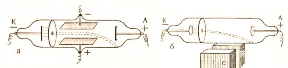
Рис. 6. Доказательство природы катодных лучей
