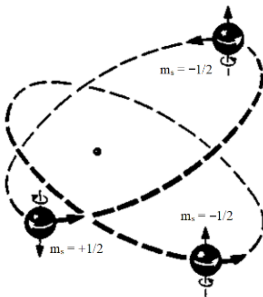
Рис. 23. Модель орбитального и собственного движения электронов как частиц в атоме лития
