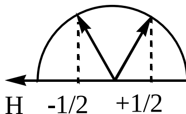
Проекции спина на выбранную (магнитную) ось
