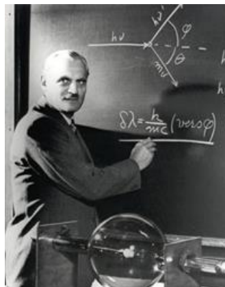
Артур Холли Комптон (1892-1962)
