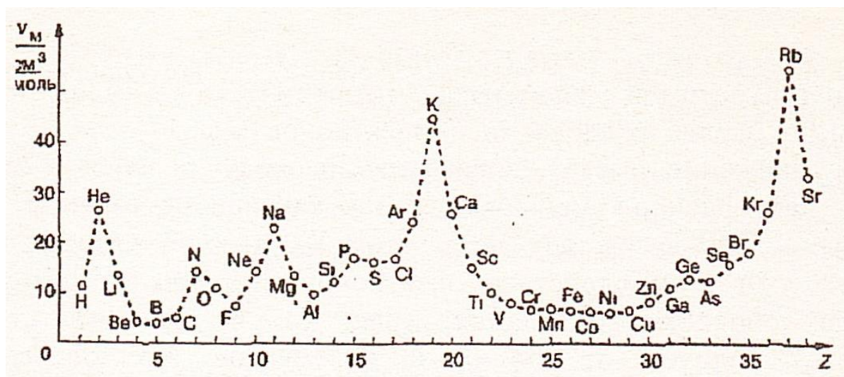
Молярные атомные объёмы элементов Таблица Мейера, 1870 г.
