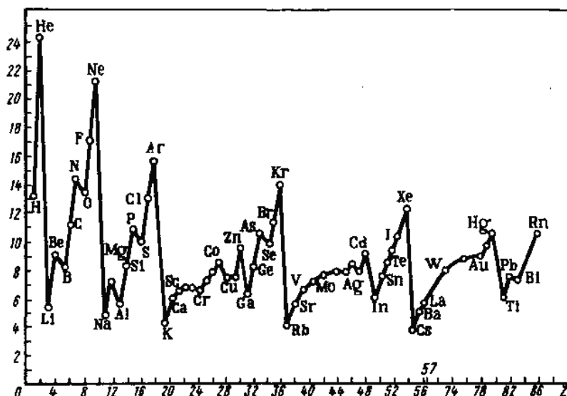
Рис. 37. Периодическая зависимость первой энергии ионизации атомов элементов (эВ) от порядкового номера Z
