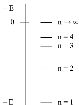
Рис. 17. Диаграмма энергетических уровней атома
