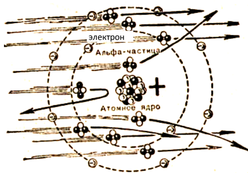
Рис. 10. Рассеивание \alpha -частиц атомным ядром
