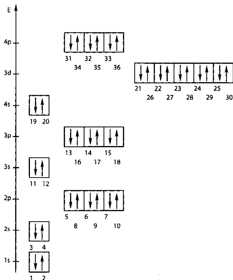
Рис. 26. Последовательность заполнения электронами энергетических уровней и подуровней, а также орбиталей в многоэлектронных атомах
