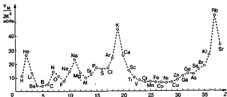
Рис. 36. Молярные атомные объёмы элементов
