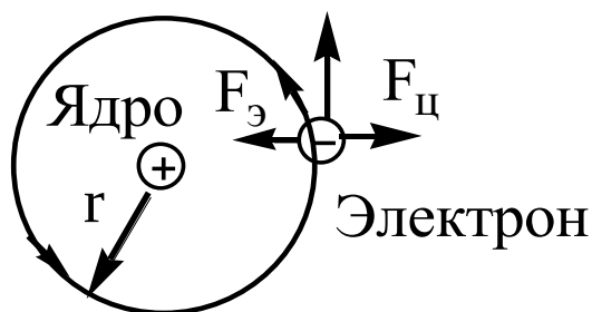
Рис. 8. Схема сил, возникающих при движении электрона в атоме водорода
