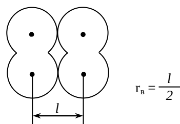
Рис. 34. Радиус атома водорода по Ван-дер-Ваальсу в молекуле водорода H_2
