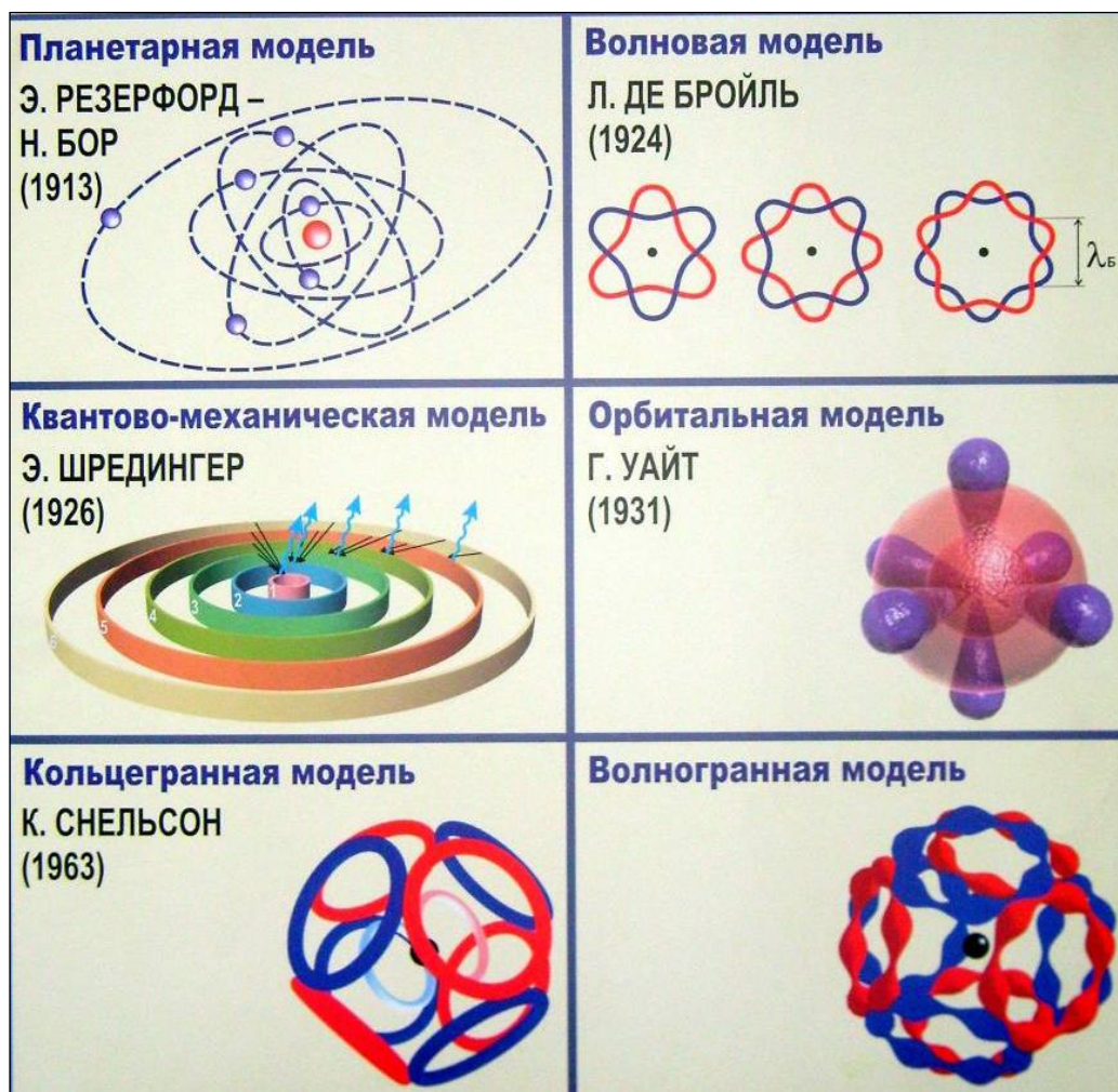
Рис. 11. Исторические и современные модели атома
