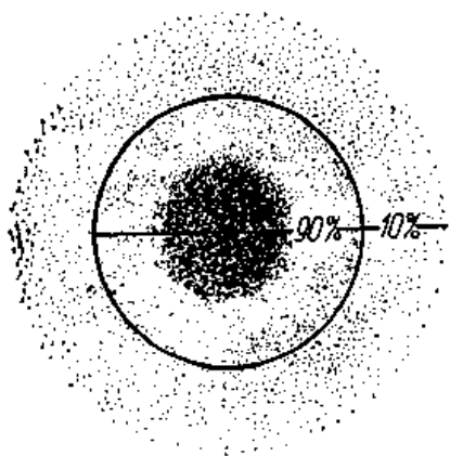
Рис. 15. Электронное облако и граница атомной орбитали в атоме водорода
