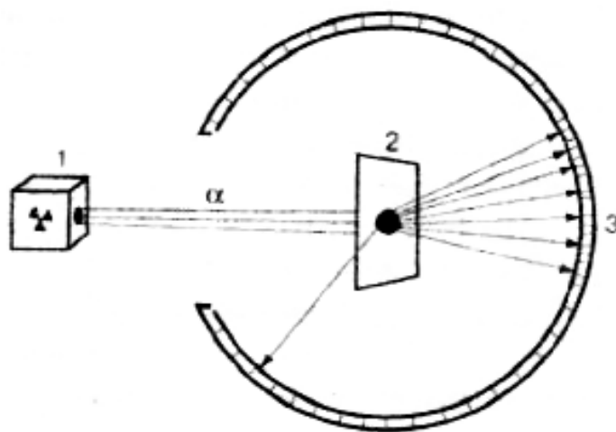
Рис. 9. Опыт Резерфорда
