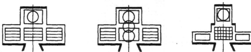
Рисунок 9. Примеры схем построения глубинной колосниковой сцены с двумя карманами и арьерсценой (варианты механического оборудования показаны условно)
