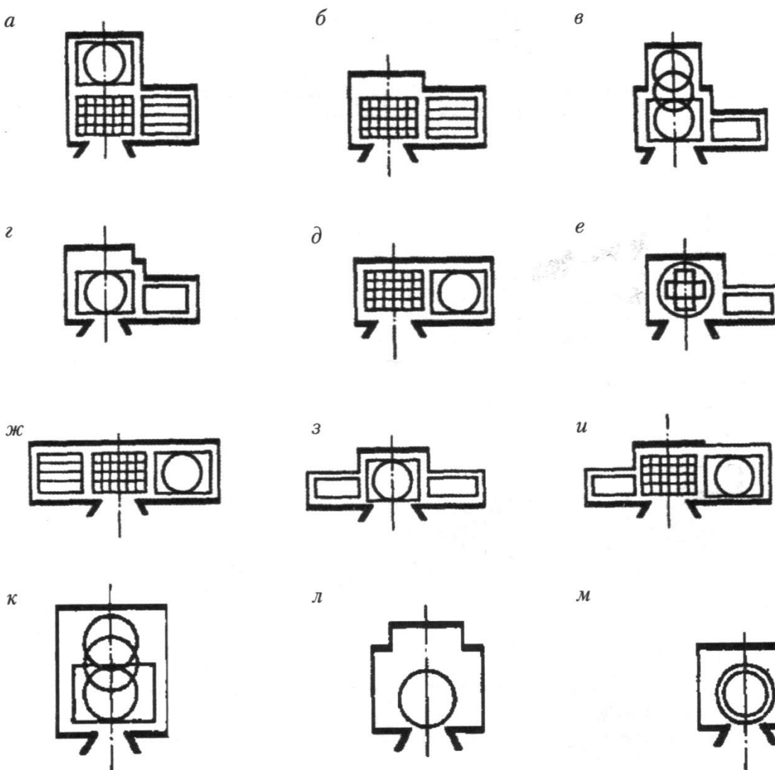
Рисунок 10. Примеры основных схем построения глубинной колосниковой сцены, карманов и арьерсцены (варианты механического оборудования показаны условно): а –
