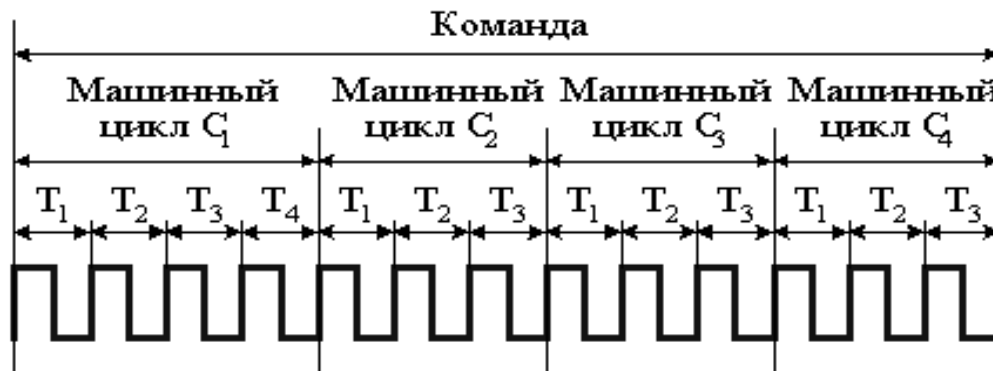
Рис. 2.1. Временная диаграмма команды LDA
