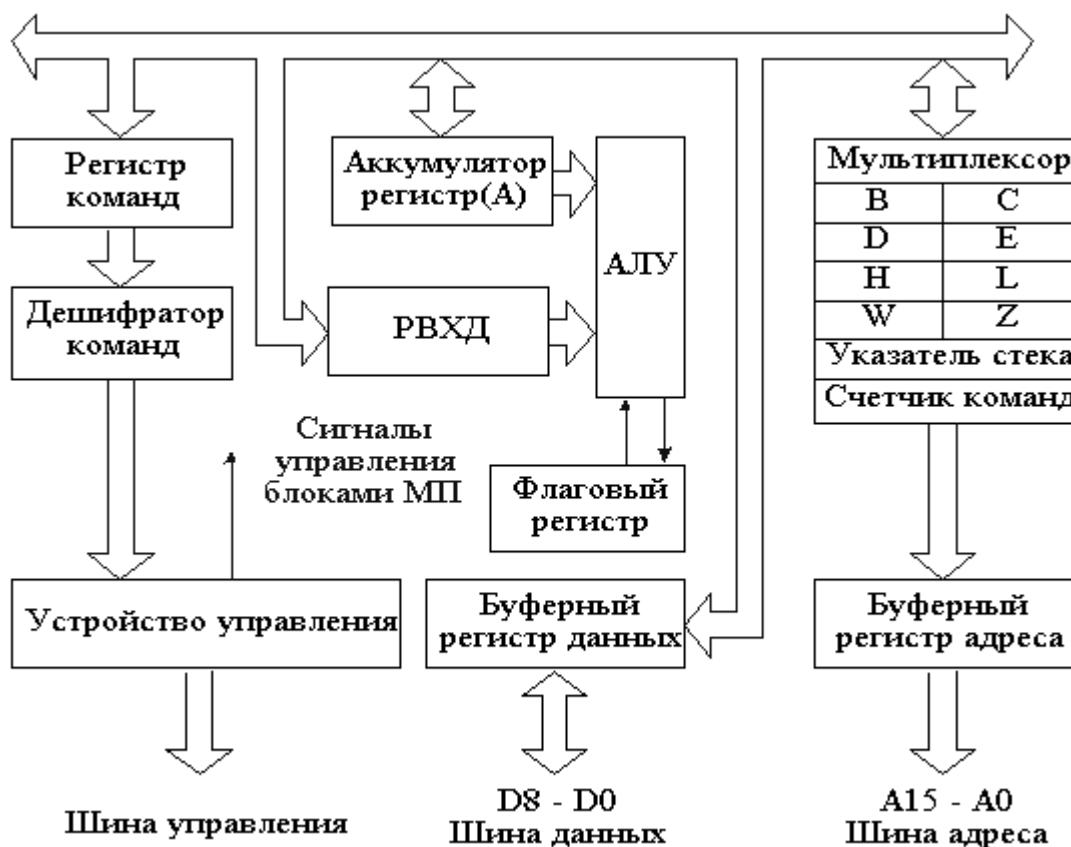
Рис. 1.1. Типовая структура микропроцессора
