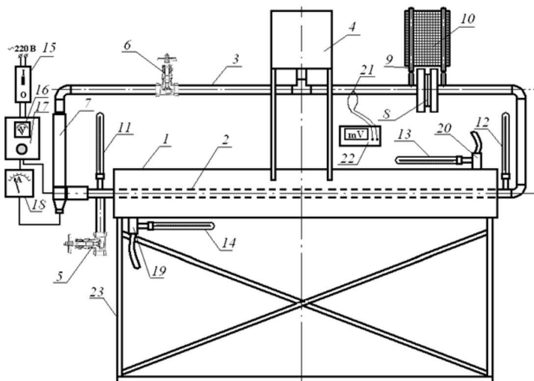
Рис. 5. Лабораторная установка для исследования работы теплообменника типа «труба в трубе»:
