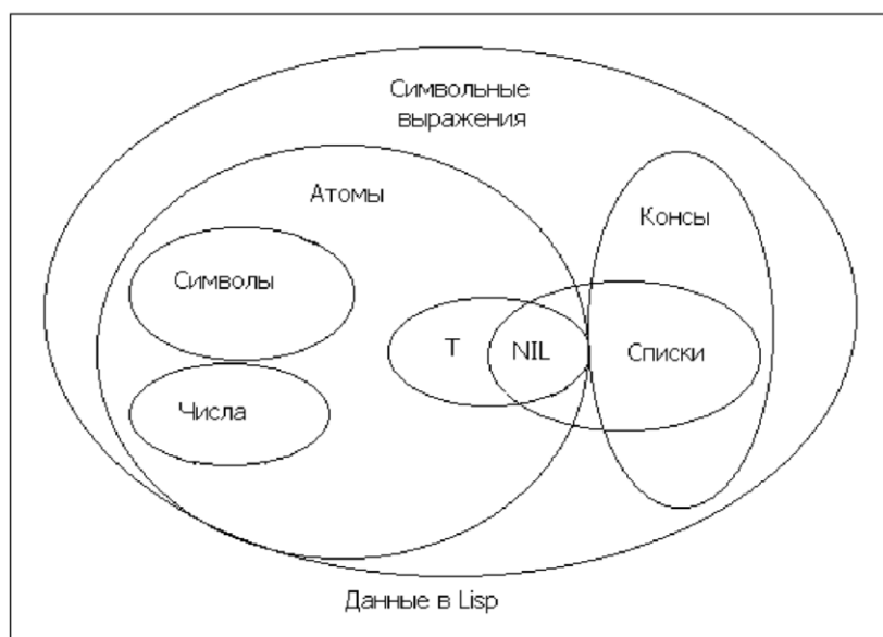
Рис. 4. Данные в Lisp
