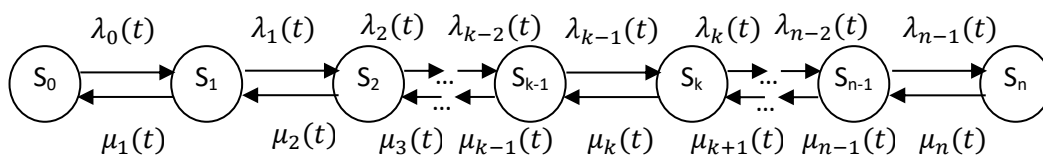
Рис. 10.4. Граф состояний для процесса гибели и размноже-
